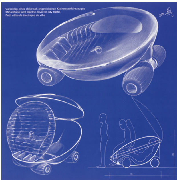
fig. 11 Luigi Colani, Vorschlag eines elektrisch angetriebenen Kleinstadtfahrzeuges , aus der Mappe VLEM , 1971, Sammlung Siekmann Berlin © Colani Design GmbH
